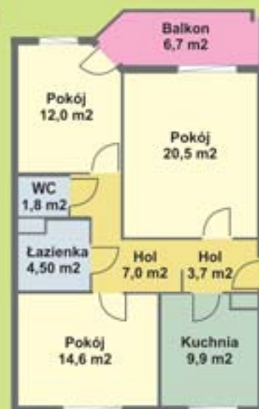
Przykładowe mieszkanie trzypokojowe 74 m 2 .
